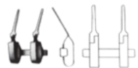
BIEMER-MÜLLER 45-115 Çene uzunluğu/Lenght of jaws.9 mm Açıklık/Opening 5 mm Kapanma kuvveti/Closing force 25-30 gr.
